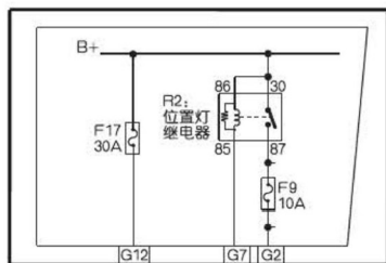
发动机舱保险丝盒
