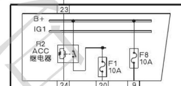
座舱保险丝盒
