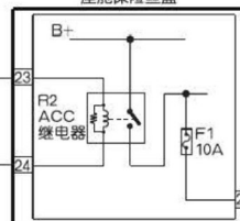
座舱保险丝盒
